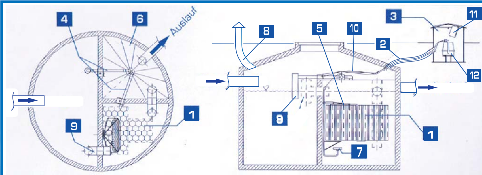
Vorklärung mit angeschlossenem Zulauf und Schlauchdurchführungen
